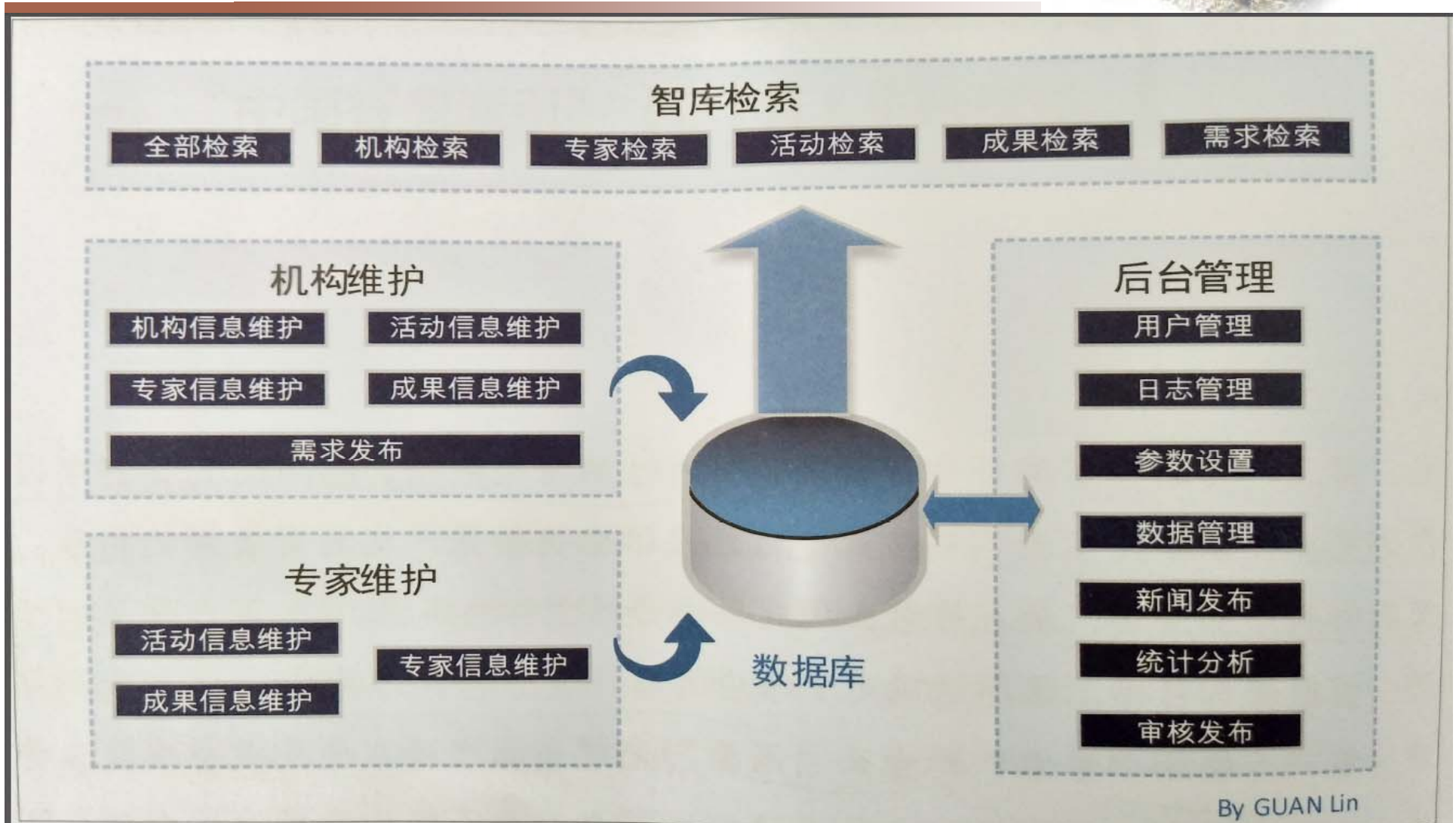
图1 CTTI框架
